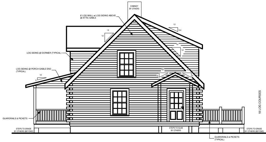
RIGHT ELEVATION
