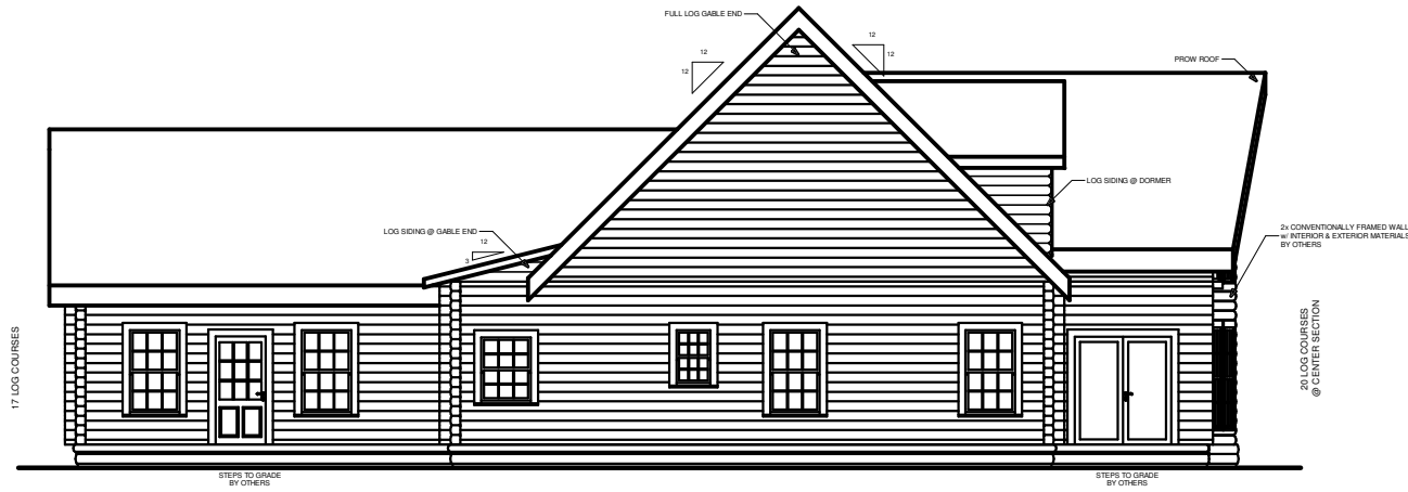
RIGHT ELEVATION
