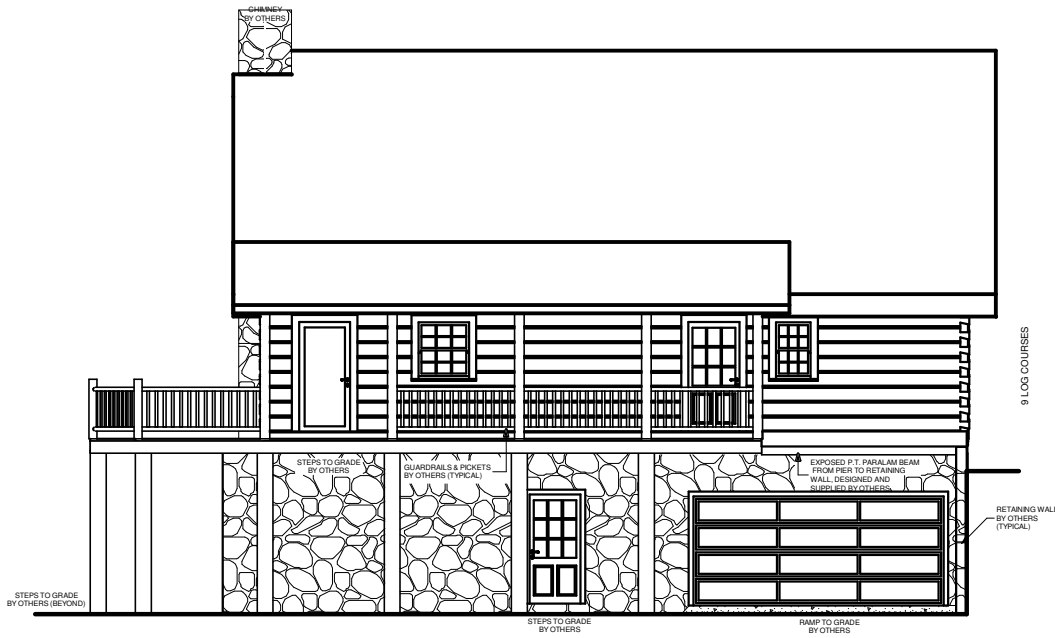
RIGHT ELEVATION
