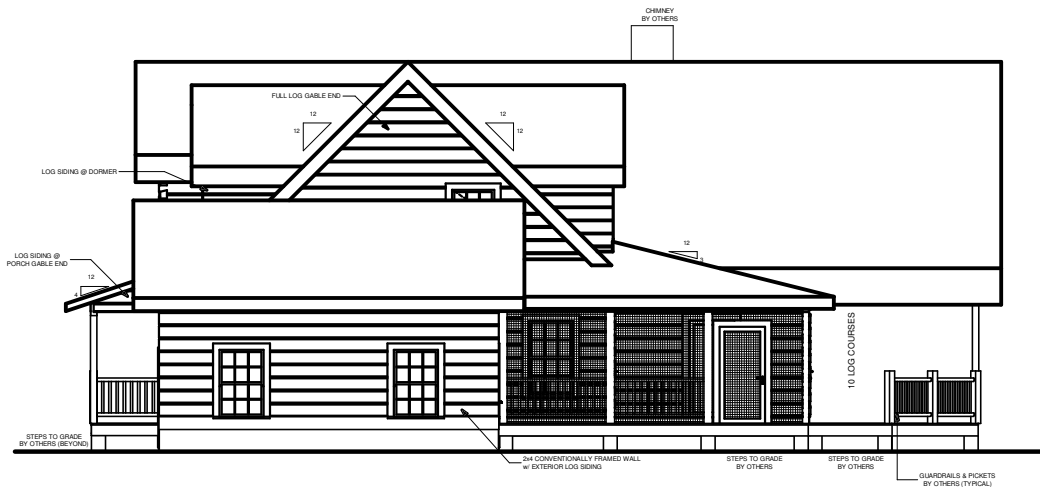
RIGHT ELEVATION
