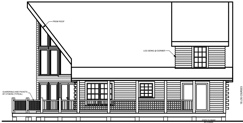
RIGHT ELEVATION
