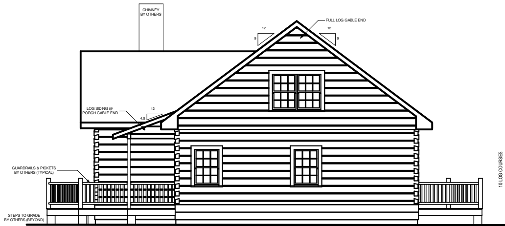
RIGHT ELEVATION
