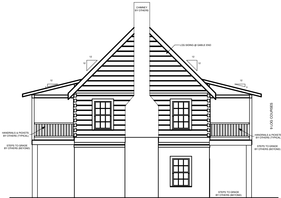
RIGHT ELEVATION
