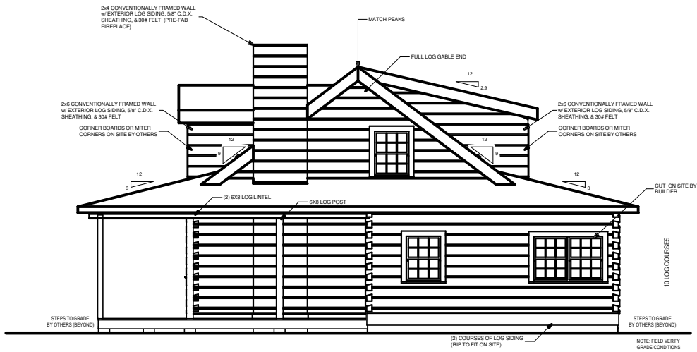
RIGHT ELEVATION
