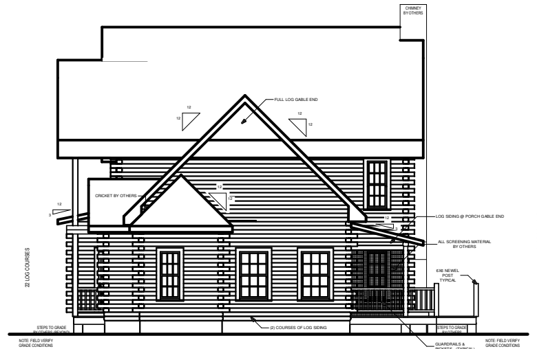
RIGHT ELEVATION
