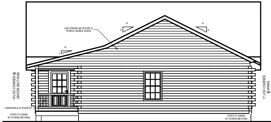
RIGHT ELEVATION
