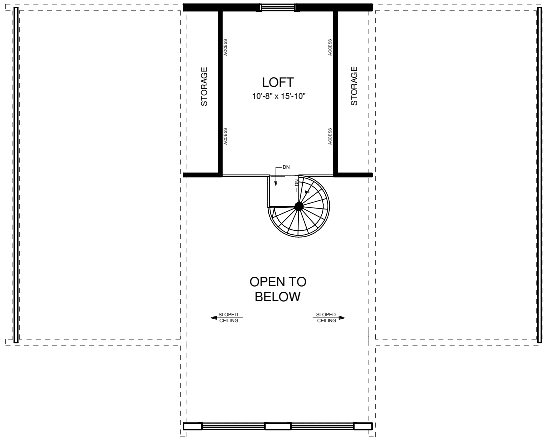
LOFT PLAN
