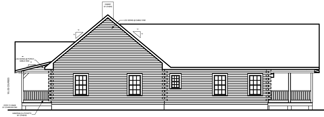
RIGHT ELEVATION
