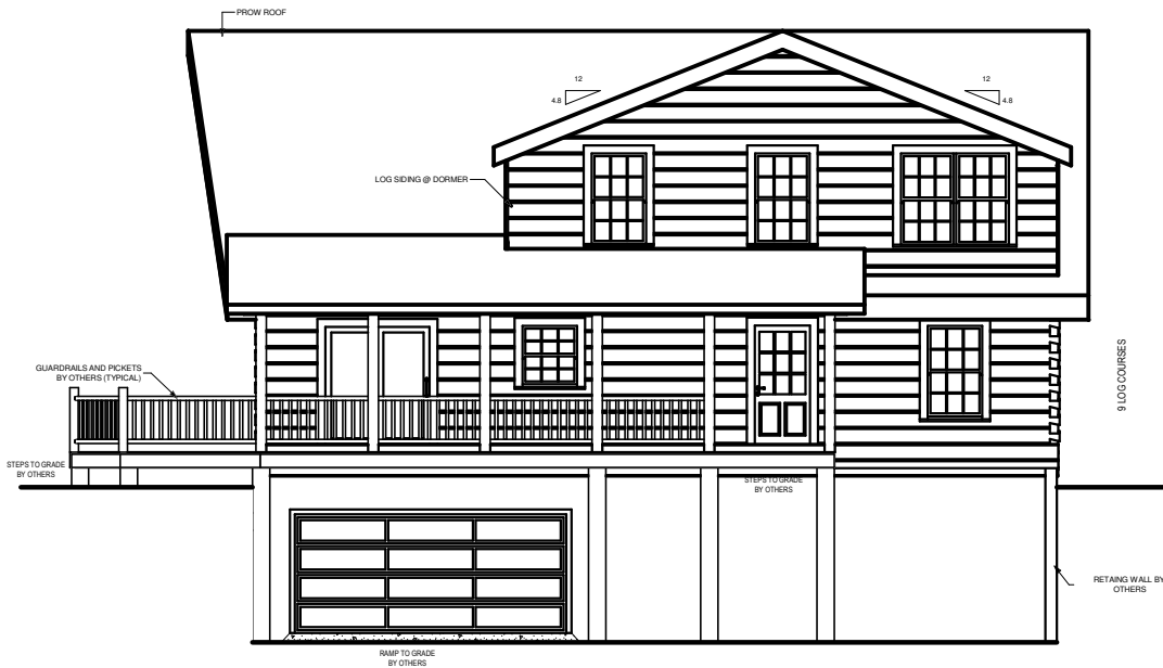
RIGHT ELEVATION
