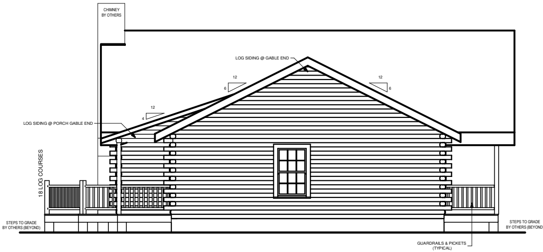
RIGHT ELEVATION
