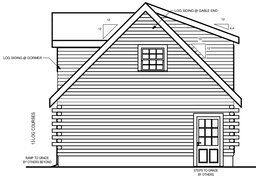
RIGHT ELEVATION
