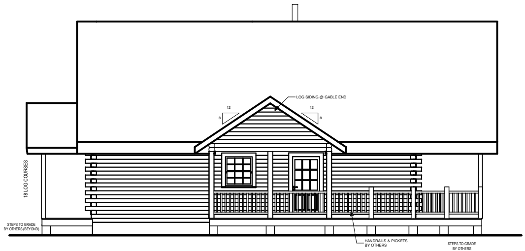
RIGHT ELEVATION
