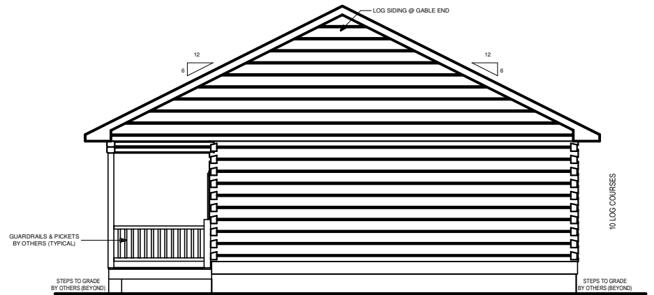
RIGHT ELEVATION
