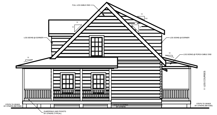
RIGHT ELEVATION
