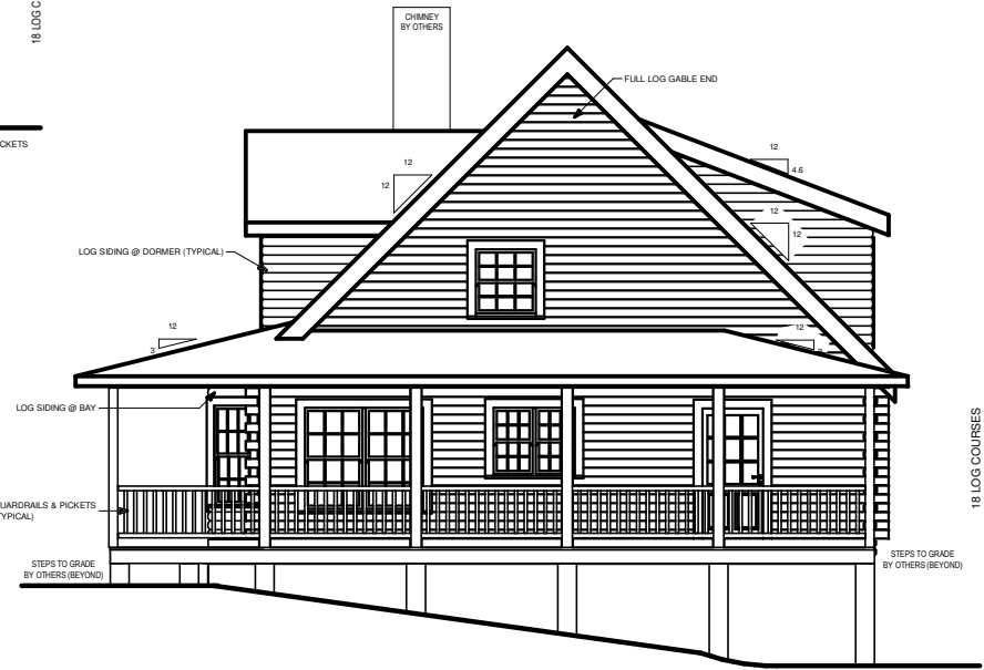
RIGHT ELEVATION
