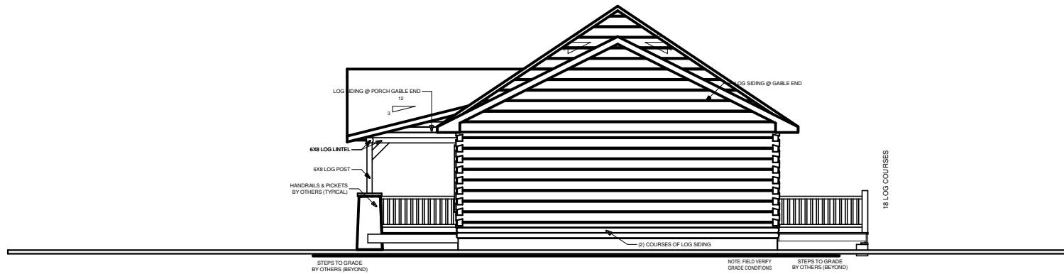
RIGHT ELEVATION
