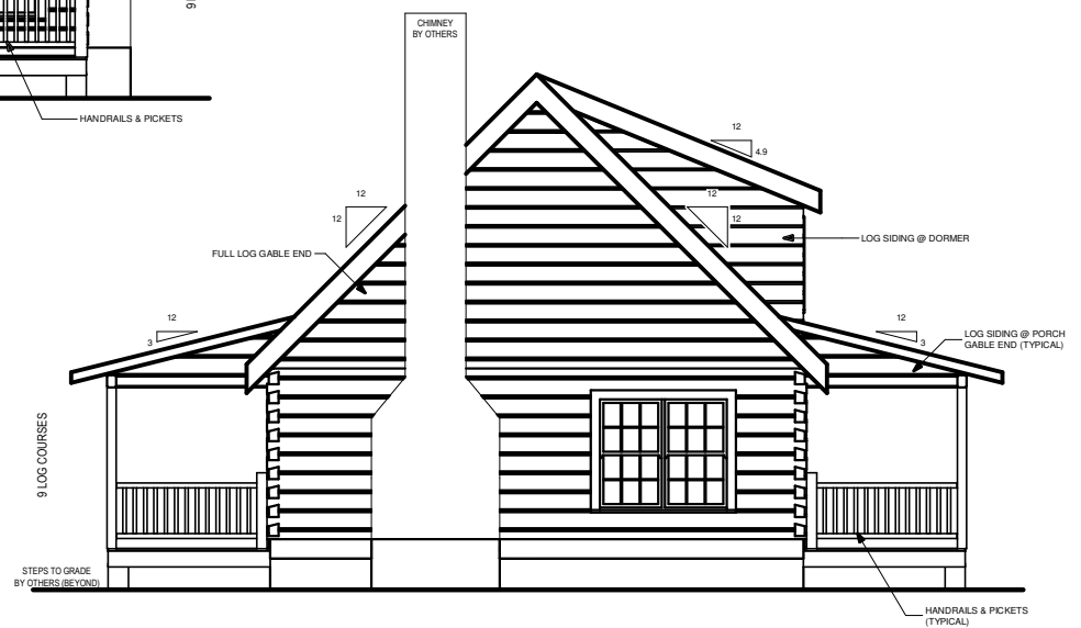
RIGHT ELEVATION
