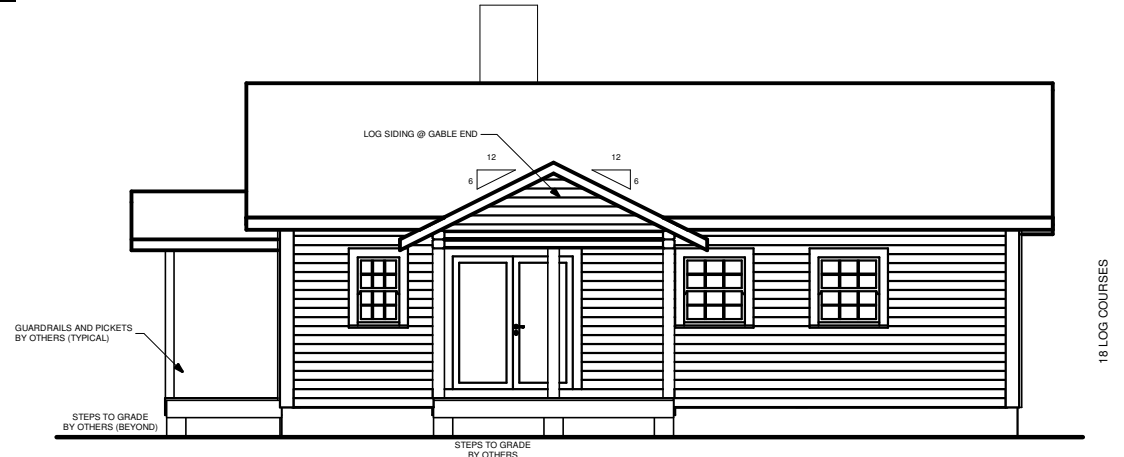
RIGHT ELEVATION
