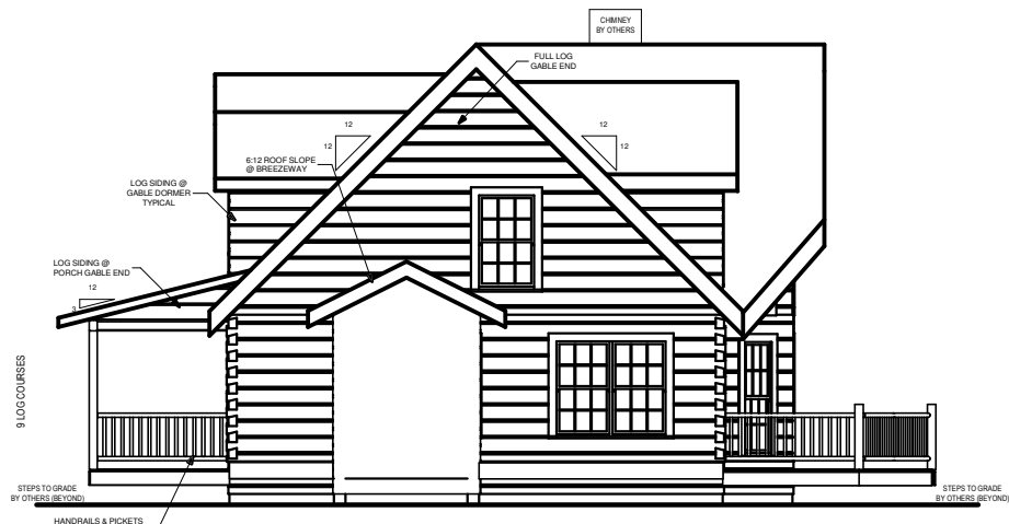
RIGHT ELEVATION
