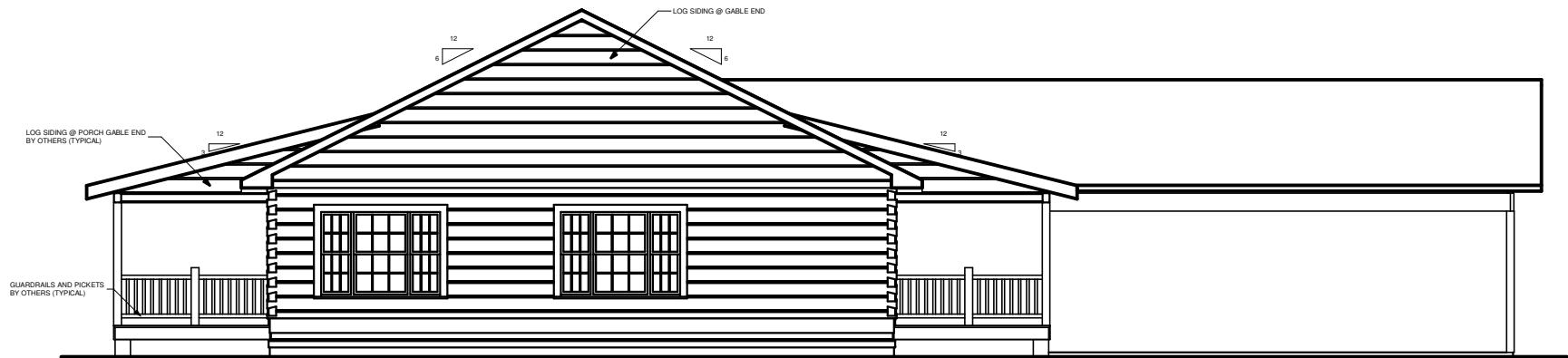
RIGHT ELEVATION
