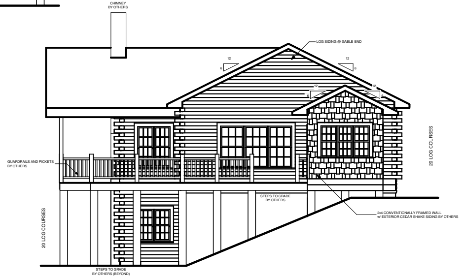
RIGHT ELEVATION
