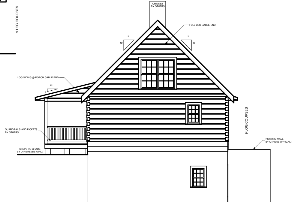
RIGHT ELEVATION
