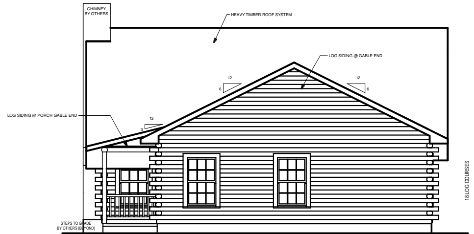
RIGHT ELEVATION
