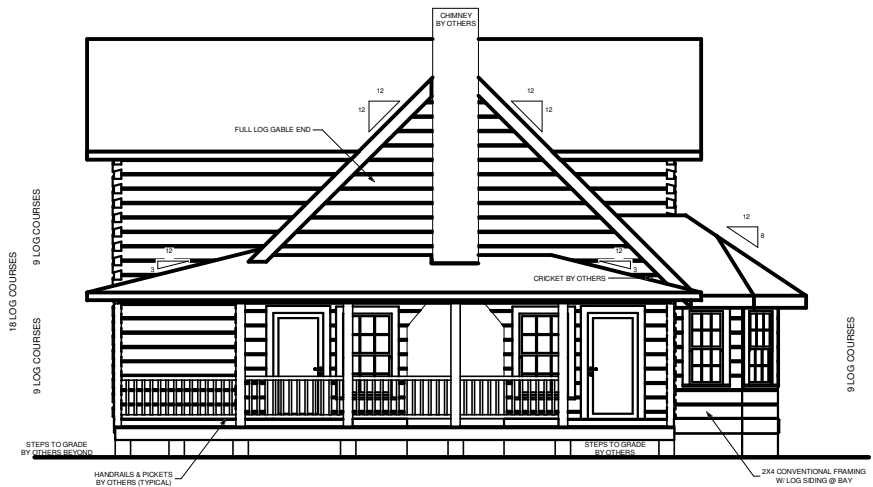
RIGHT ELEVATION
