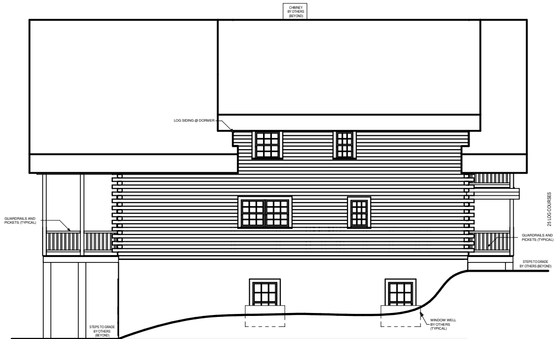
RIGHT ELEVATION
