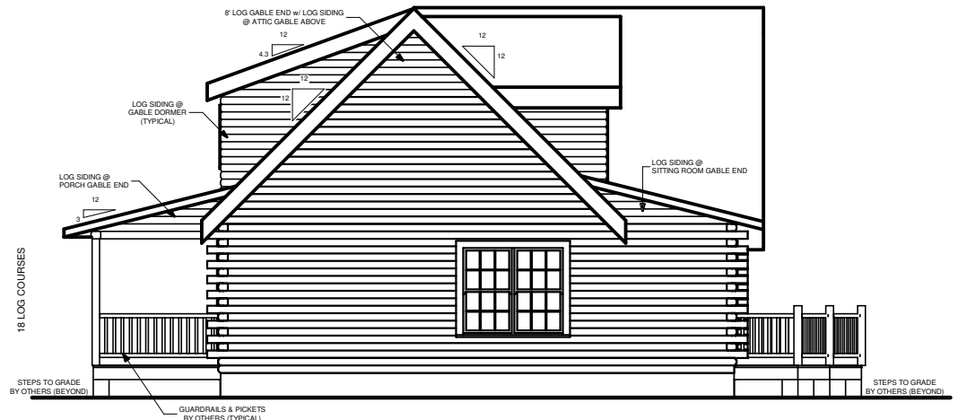
RIGHT ELEVATION
