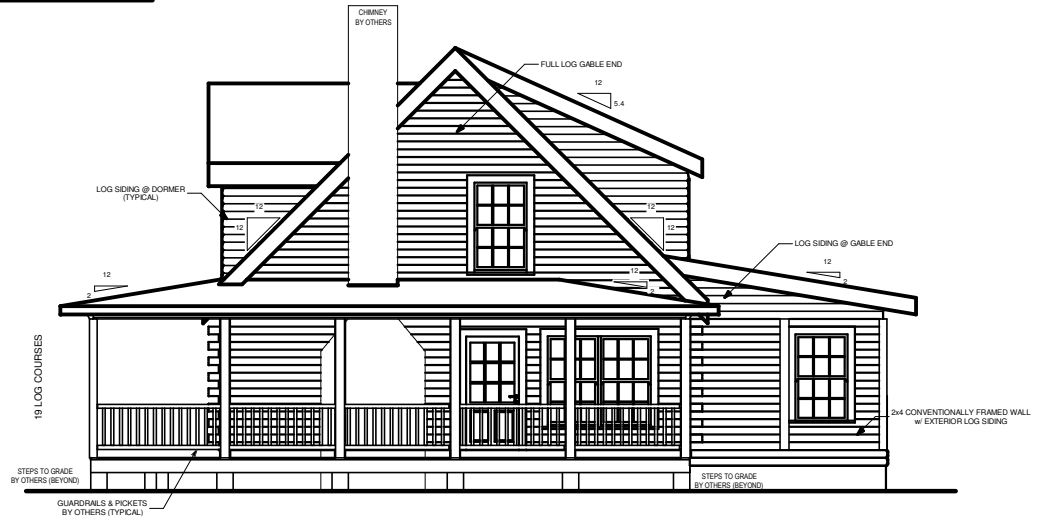
RIGHT ELEVATION
