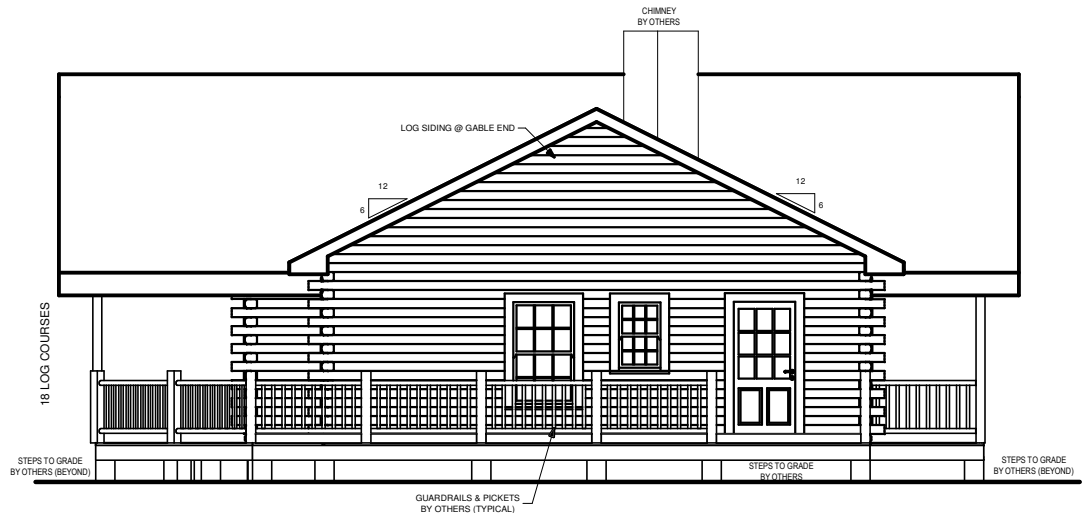
RIGHT ELEVATION
