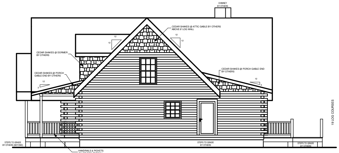
RIGHT ELEVATION
