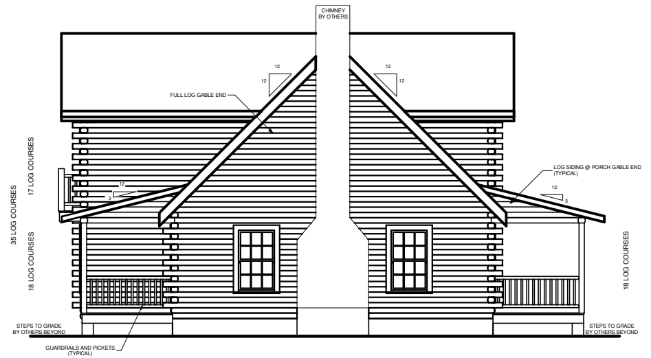
RIGHT ELEVATION
