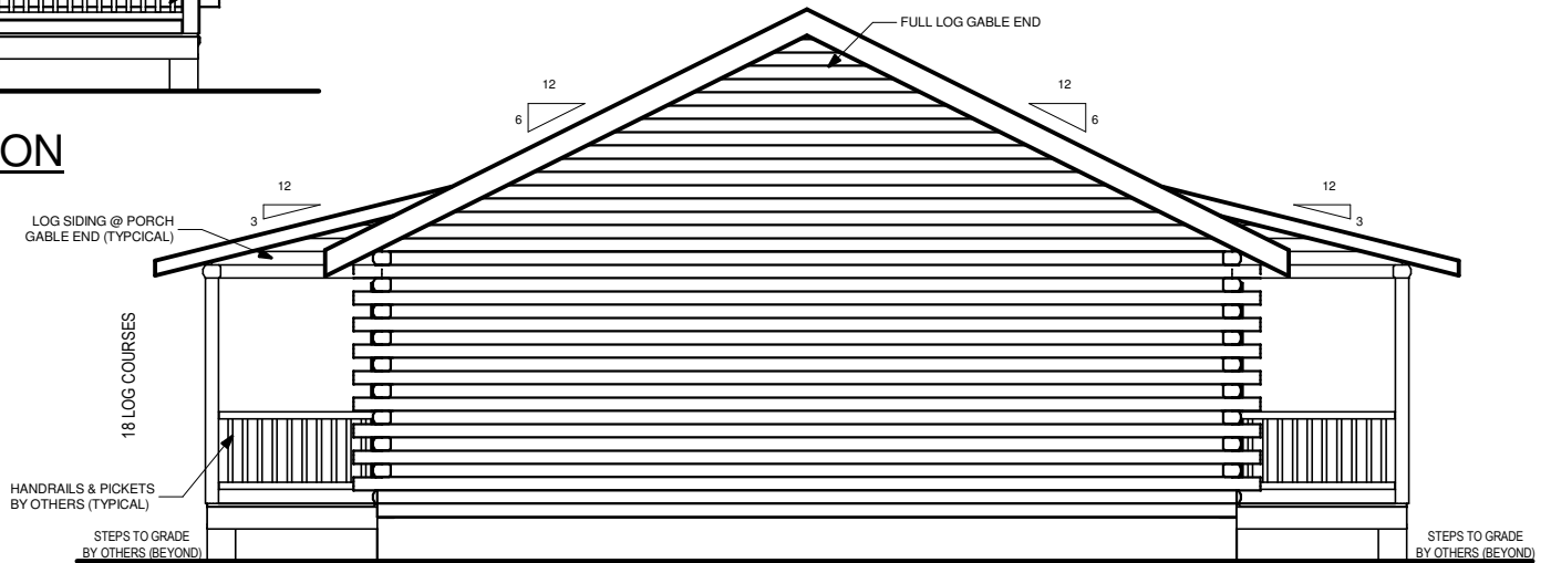
RIGHT ELEVATION
