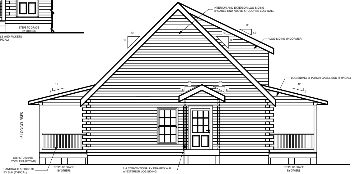
RIGHT ELEVATION
