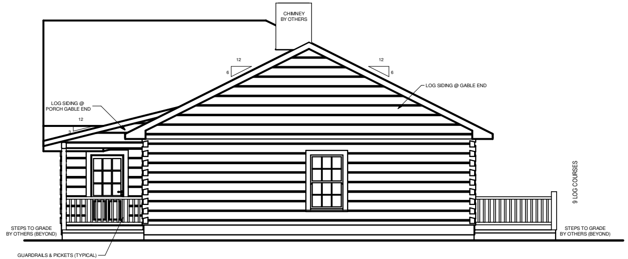
RIGHT ELEVATION
