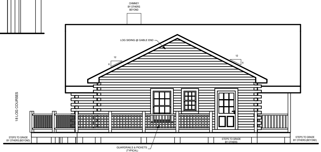
RIGHT ELEVATION
