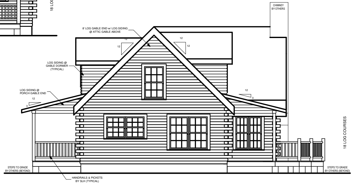
RIGHT ELEVATION
