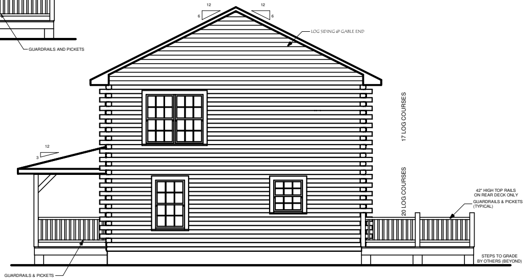
RIGHT ELEVATION
