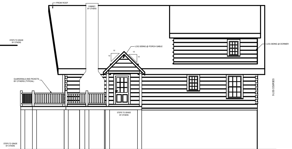
RIGHT ELEVATION
