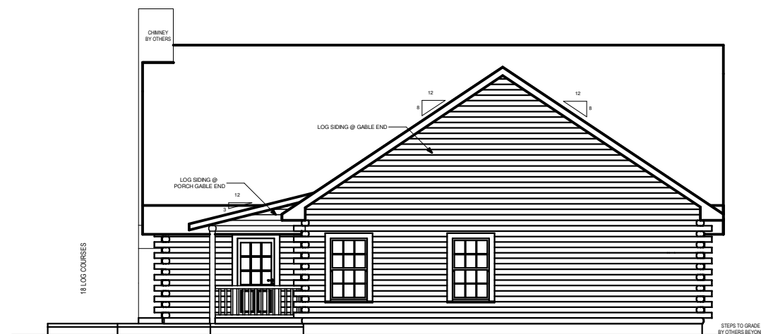
RIGHT ELEVATION
