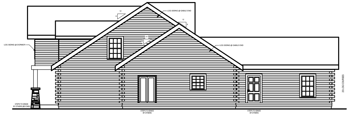
RIGHT ELEVATION
