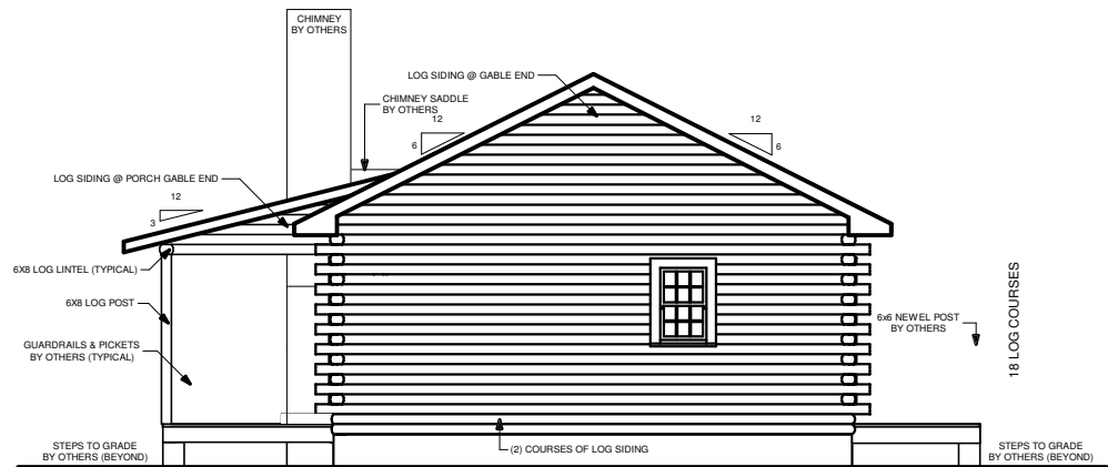
RIGHT ELEVATION
