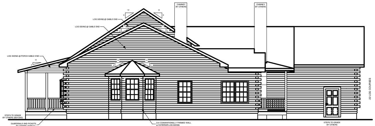
RIGHT ELEVATION
