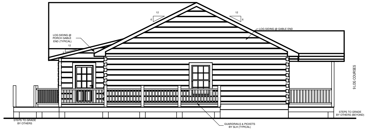
RIGHT ELEVATION
