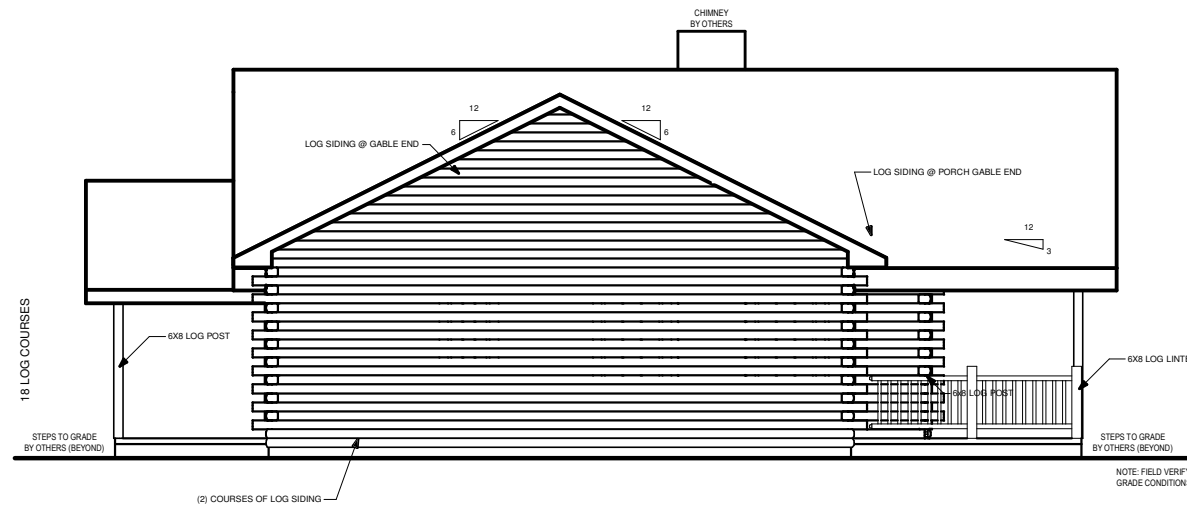
RIGHT ELEVATION
