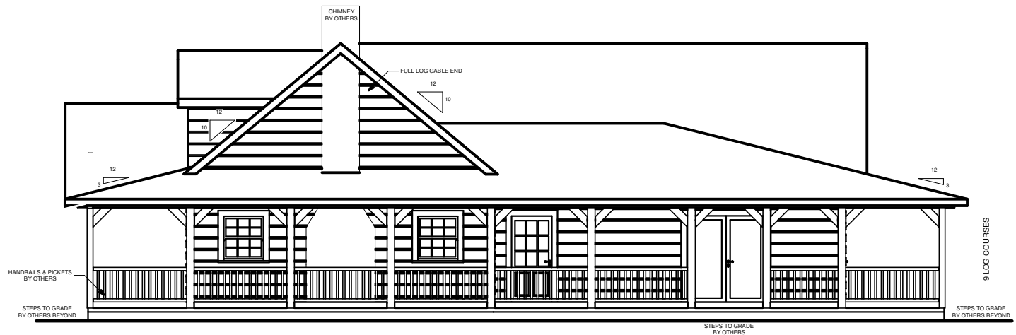
RIGHT ELEVATION
