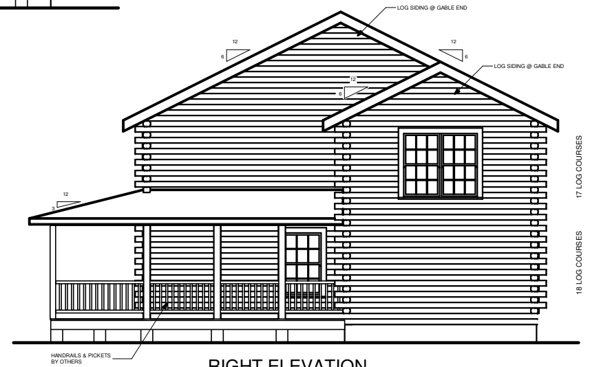
RIGHT ELEVATION
