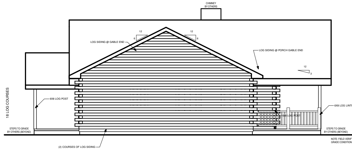
RIGHT ELEVATION
