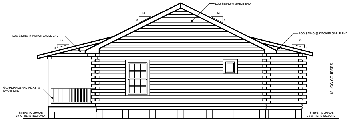
RIGHT ELEVATION
